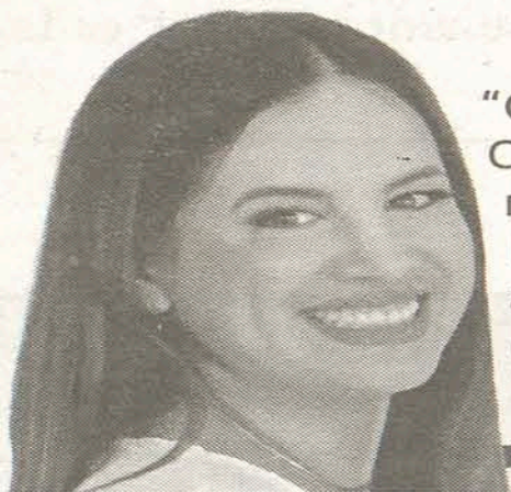
Ana Luiza Folchini
